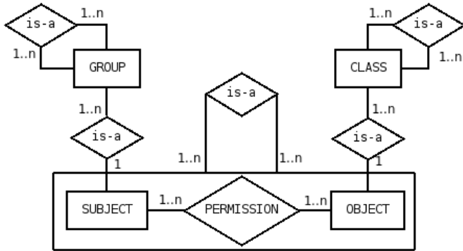
Fig. 1. The ER Diagram of the RelBAC Model.
